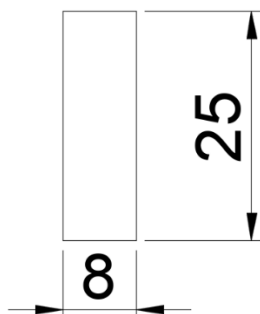
Figura 6. Secció bigueta de fusta.
