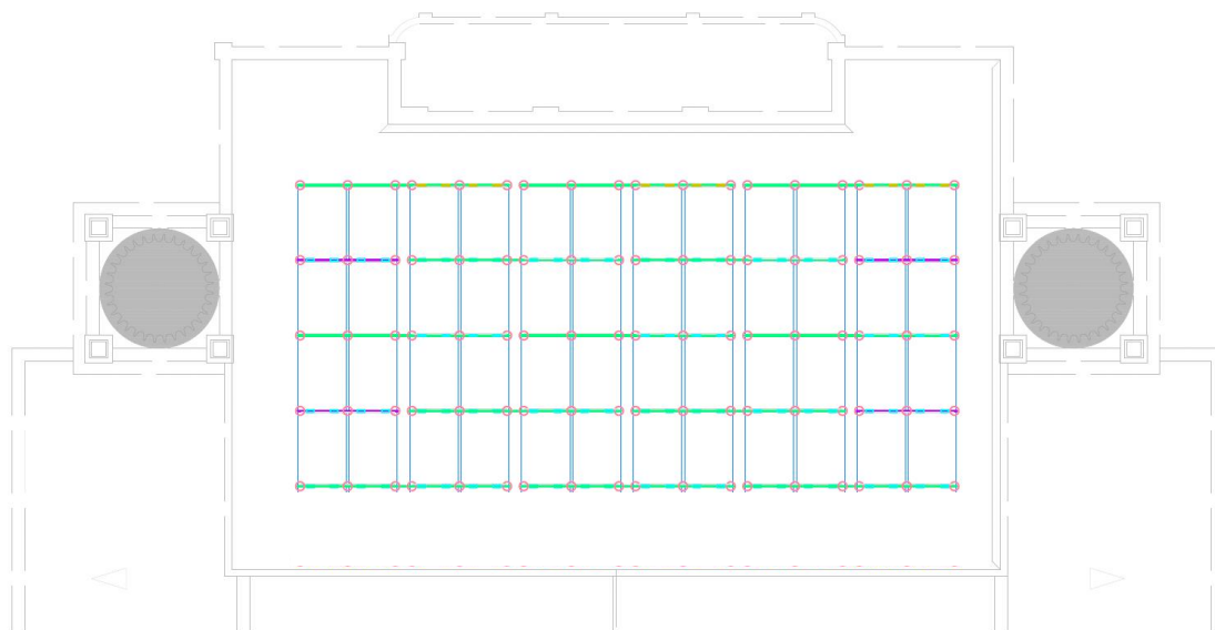
Figura 3. Plànol de l'estructura metàl·lica dels panells fotovoltaics.
