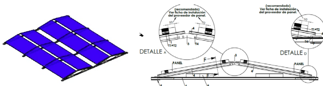
Fig. 8. Estructura inclinada Est-Oest
