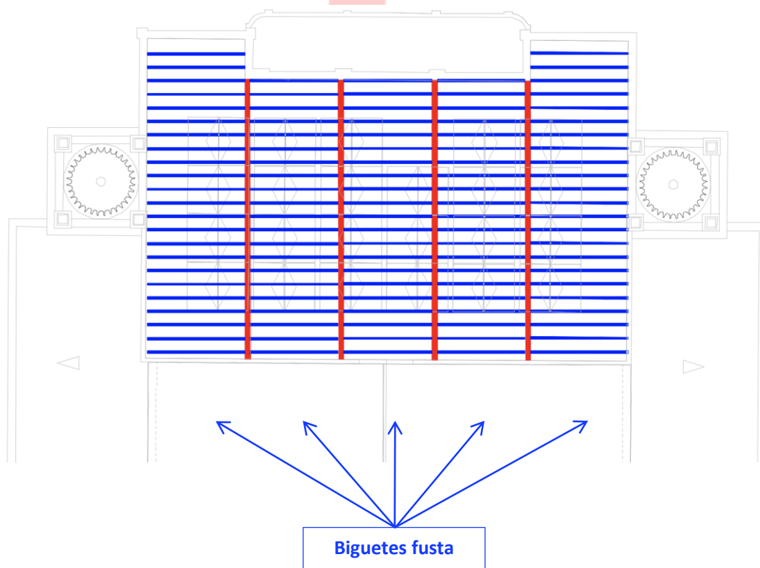
Figura 5. Estructura coberta actuació (biguetes).
