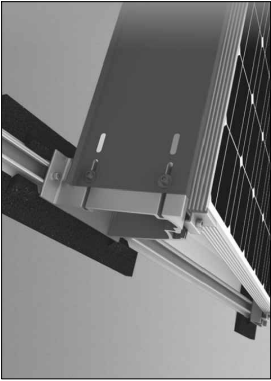
Deflectors posteriors contra la resistència del vent (Font: K2 Systems)
