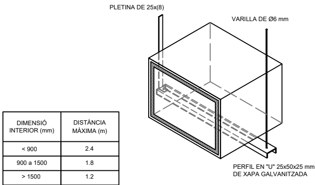
DETALL DE SUPORT DE CONDUCTES FLEXIBLES
