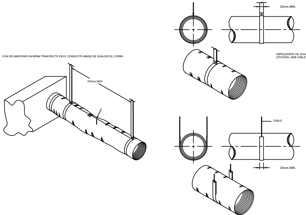
DETALL DE SUPORT DE CONDUCTES FLEXIBLES
