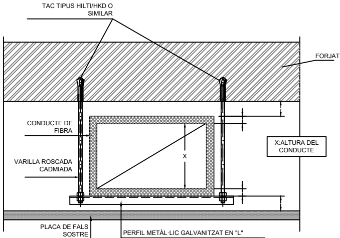
DETALL COL·LOCACIÓ DE CONDUCTE DE FIBRA EN FALS SOSTRE
