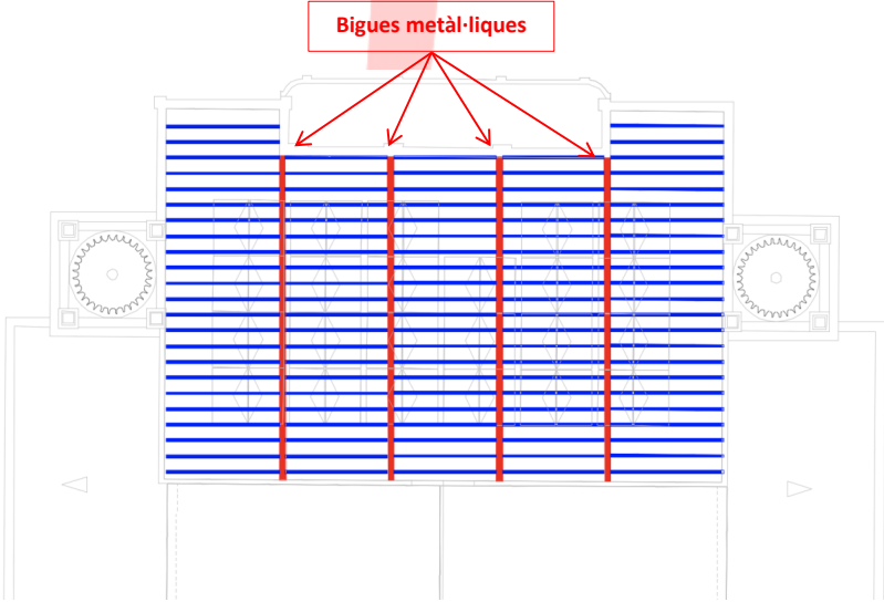
Figura 7. Estructura coberta actuació (bigues).
