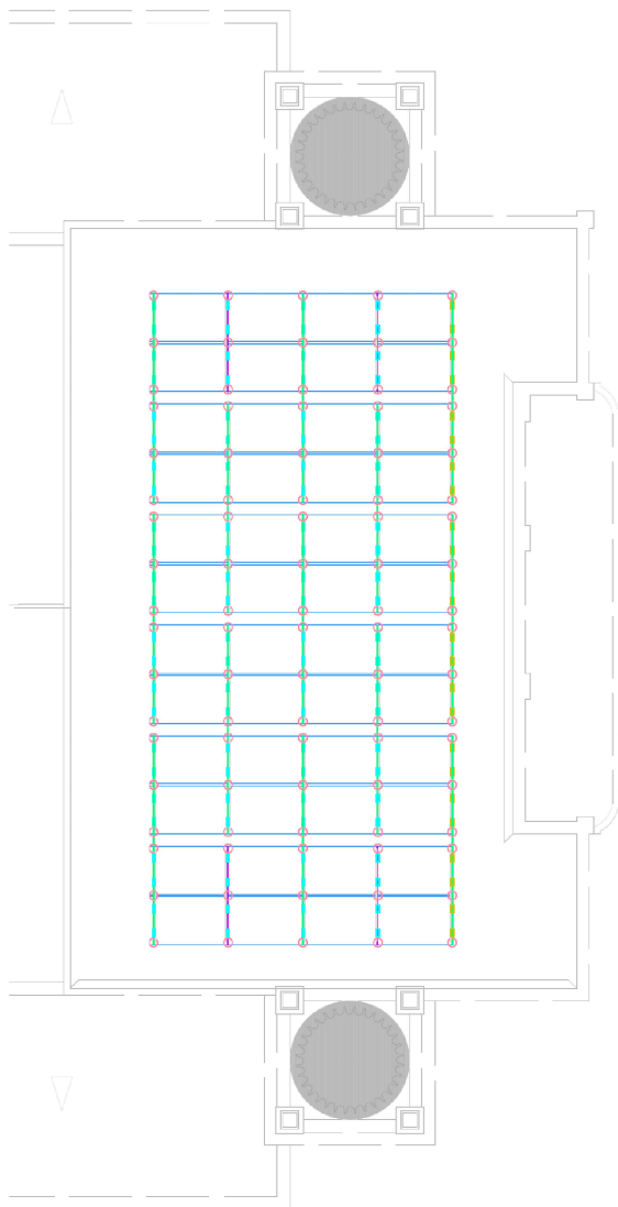
PLANTA E | 1:100
