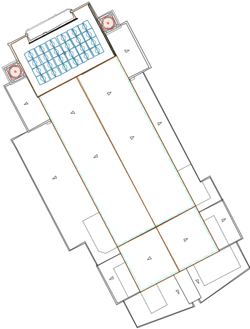
Figura 2. Plànol de la coberta amb els panells fotovoltaics.
