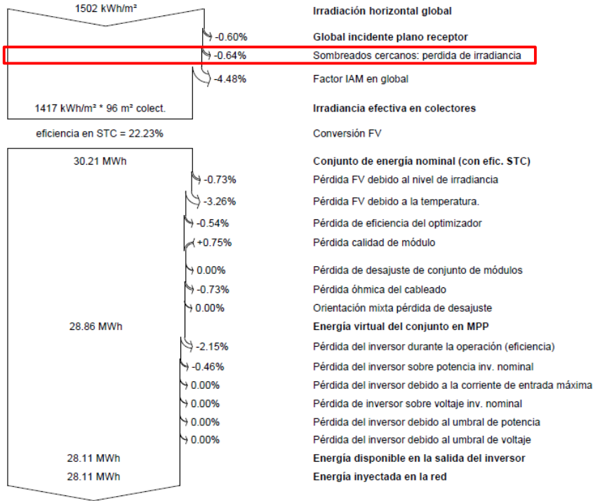
Fig. 6. Resultats de la simulació per ombres anual
