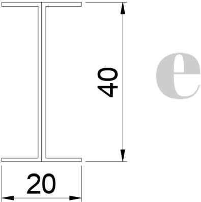
Figura 8. Secció bigueta de fusta.
