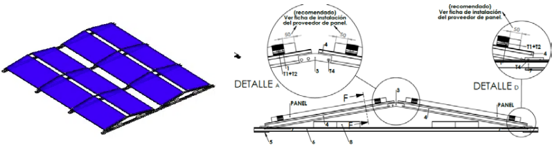
Fig. 8. Estructura inclinada Est-Oest
