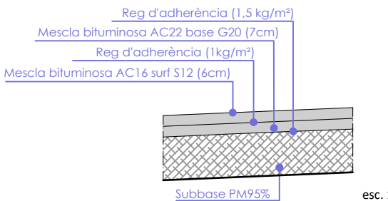
Detall Calçada
