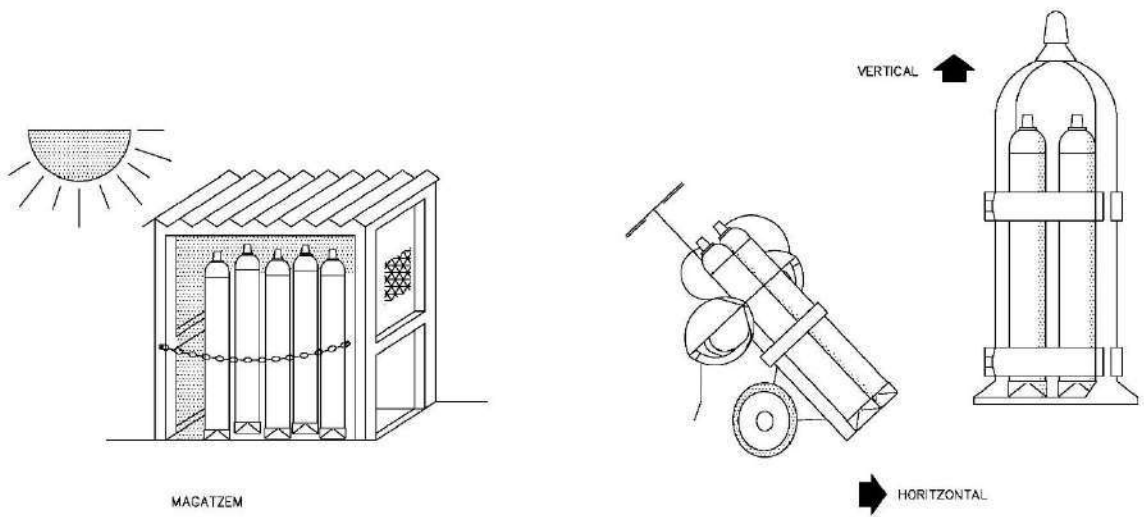
GRUP OXITALL AMB DOBLE VÀLVULA ANTIRRETORN
