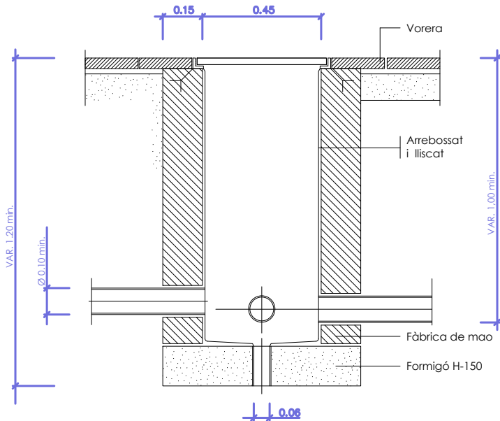
ARQUETA TIPUS
