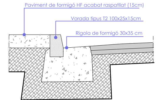
Detall vorera de formigó armat raspatllat
