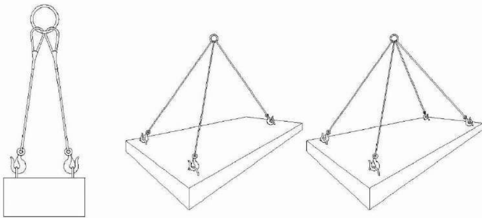
Cargues Horizontals (Precaucions a tindre hem comta per tenir-les ben subjectes)
