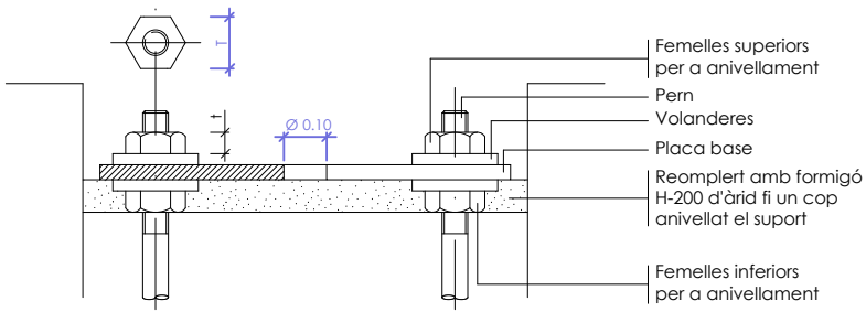
Detall ancoratges de les columnes i bàsculs
