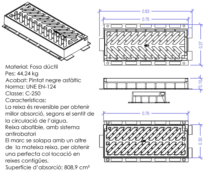
Reixa d'embornal
