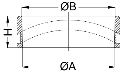
Detall clip elastomèric de connexió
