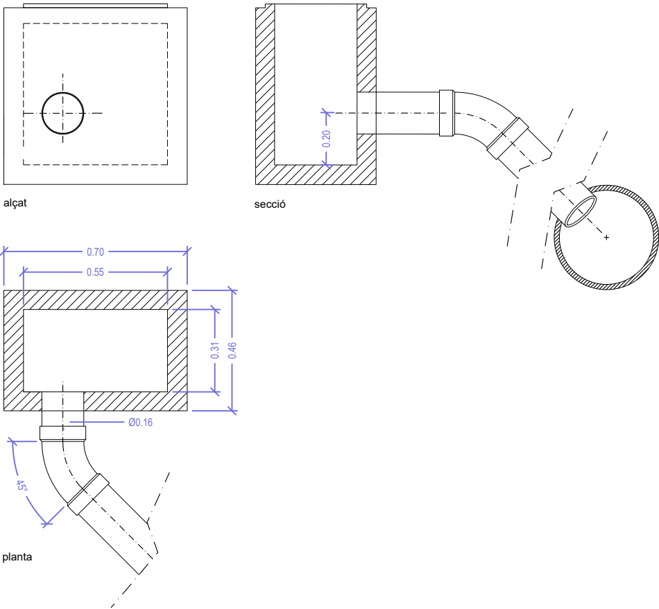
Detall embornal tub Ø160 i caixó petit
