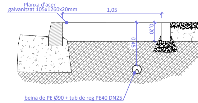
Detall escocell
