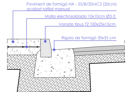
Detall vorera de formigó armat raspatllat
