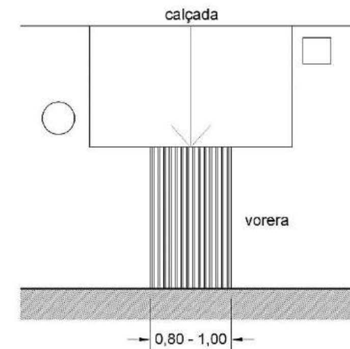
Figura 2a.5. Encreuament amb gual 120
