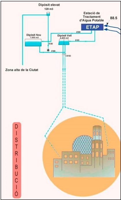
Imatge 5 i 6. Esquemes de les xarxes bàsica i secundària del Municipi de Figueres
